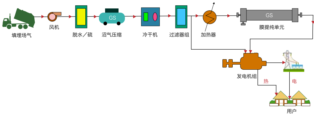
填埋场沼气发电工艺流程图
