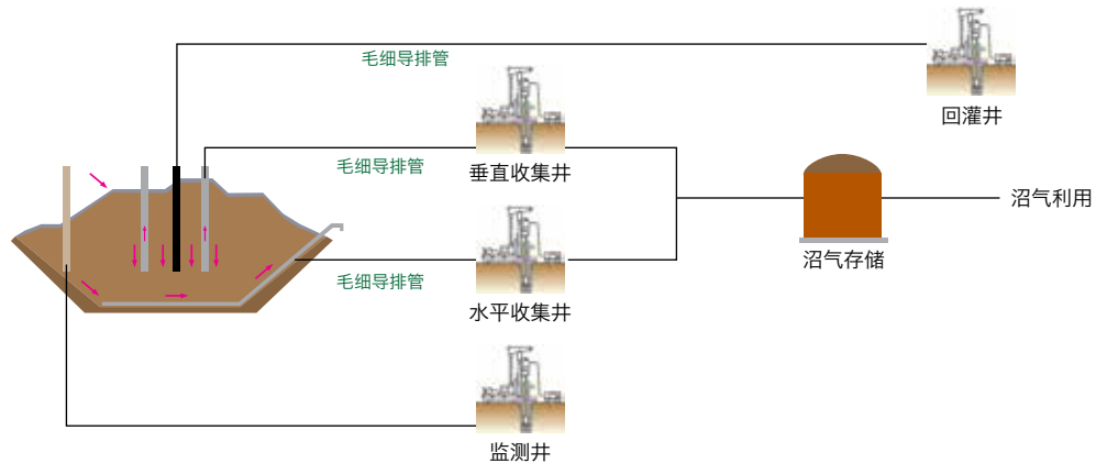
垂直+水平+毛细导排工艺流程图
